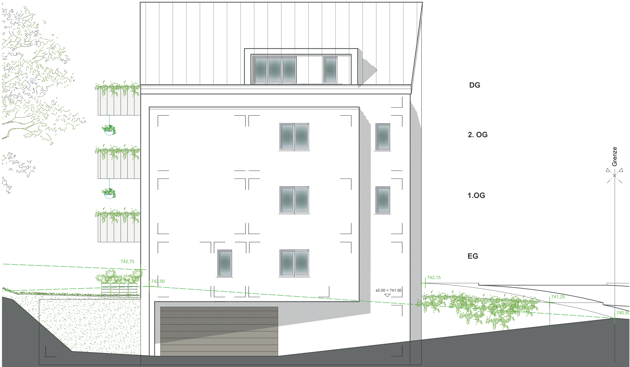
ANSICHT SÜDOST
