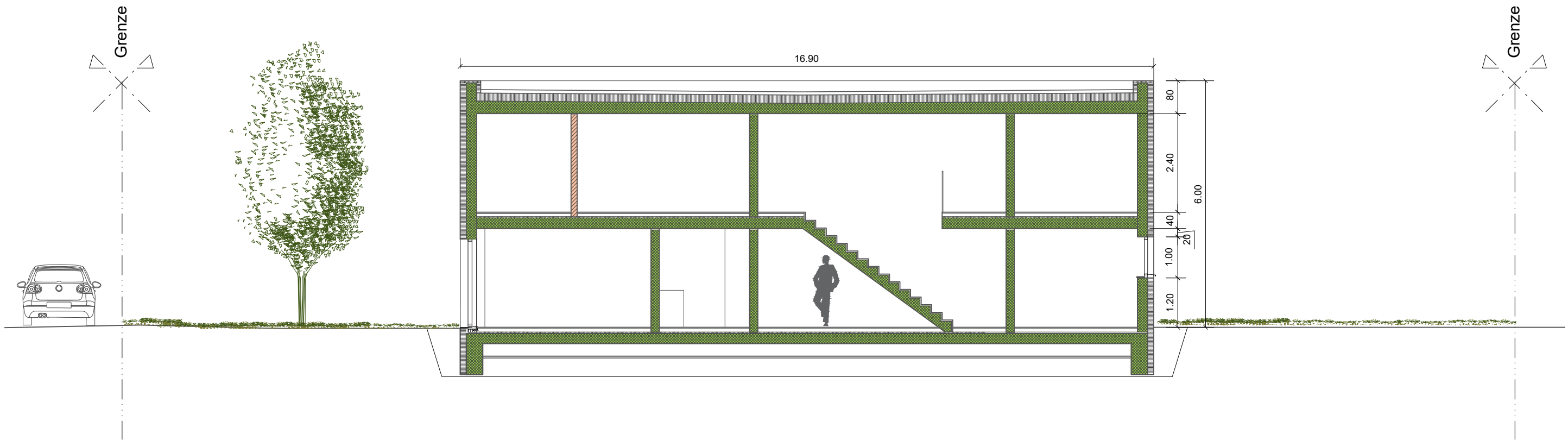
SCHNITT
